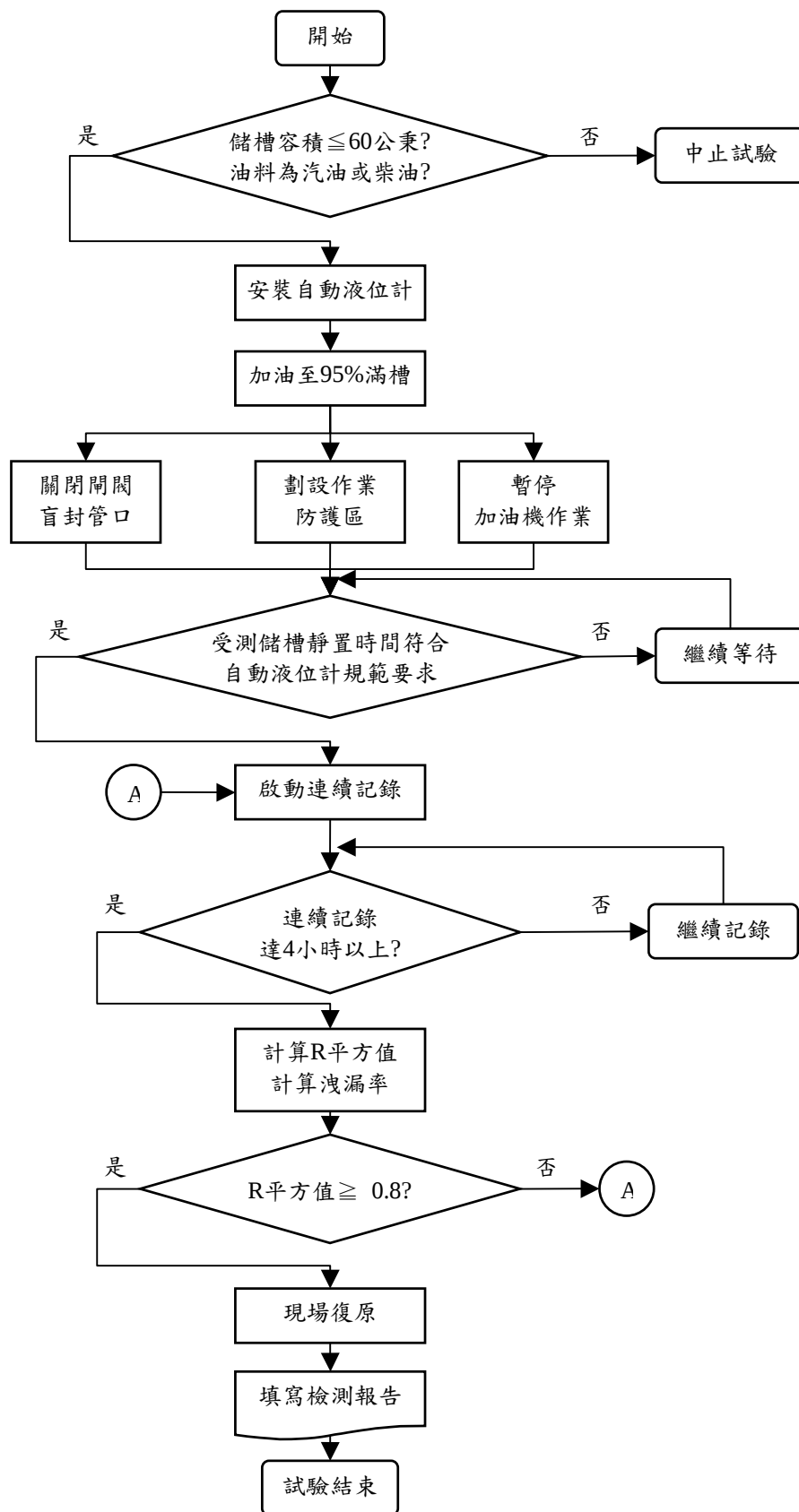
圖一 自動液位測漏作業流程
