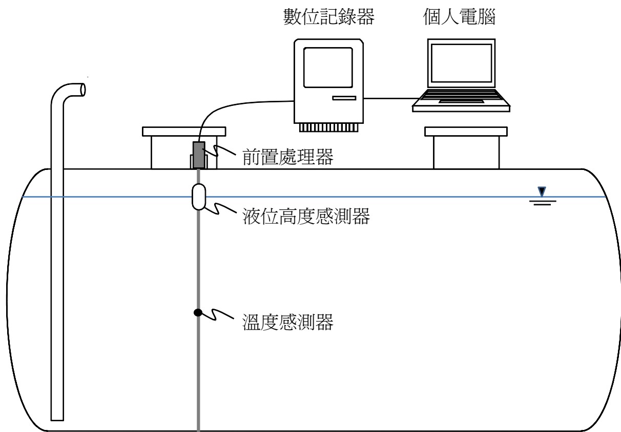
圖二 自動液位計安裝示意圖
