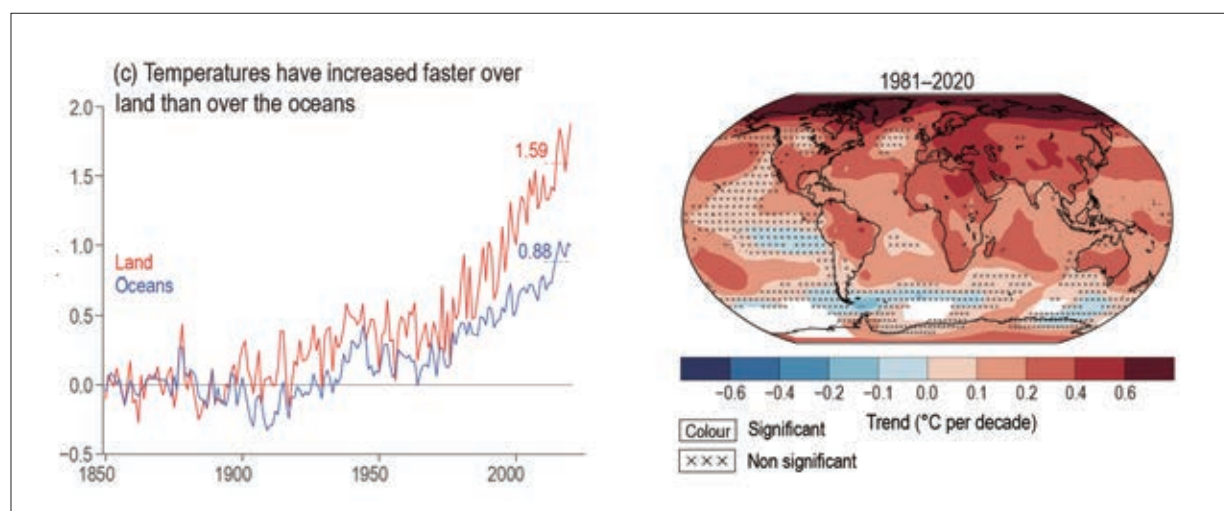
圖1.2.2 (左圖) 1850年至2020年的地表溫度距平，藍、紅線分別表示海洋與陸地溫度，並標示出最後10年的升溫數值 (摘自IPCC AR6, WGI, Figure 2.11)。(右圖) 1981年至2020年期間HadCRUTv5每10年的地表溫度趨勢 ( ^{\circ}\text{C decade}^{-1} )，x區域表示不顯著。(摘自IPCC AR6, WGI, Cross-Section Box TS.1, Figure 1)
