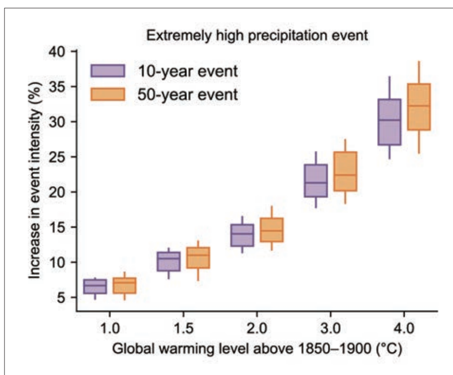
圖1.4.5 CMIP6模式在全球陸地區域。相對於1850年至1900年的GWL 1°C、GWL 1.5°C、GWL 2°C、GWL 3°C 和GWL 4°C (橫軸)，年最大日降雨量 (代表極端降水事件強度)，在10年 (紫色) 和50年 (橙色) 事件重現值的推估變化率 (縱軸)。方框中水平線與上下框線分別代表所有模式模擬的變化率的中位數與66%的不確定性範圍，而盒鬚圖上下界間距代表90%的不確定性範圍。(摘自IPCC AR6, WGI, Figure 11.15)
