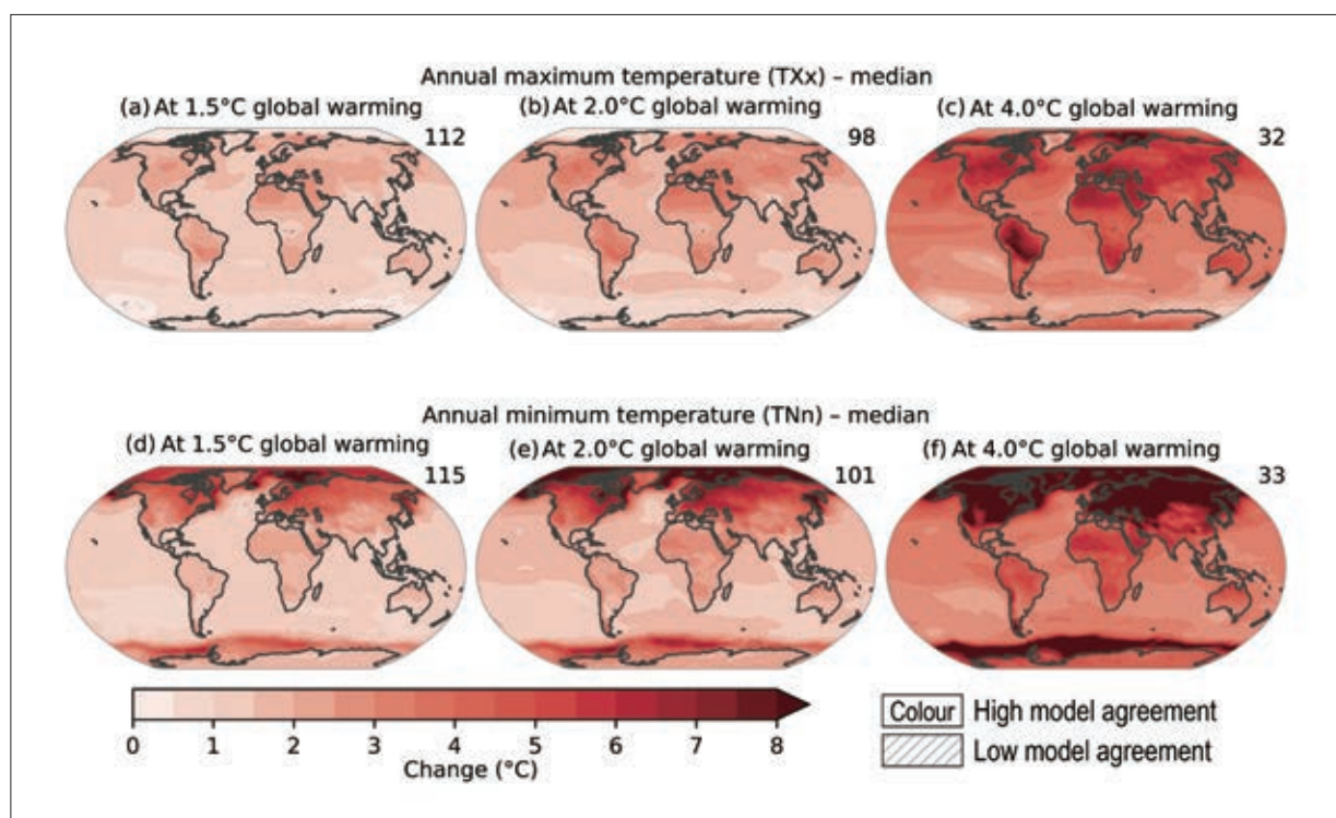
圖1.4.2 極端溫度指標之未來推估結果。(a至c) 分別為GWL 1.5°C、GWL 2°C和GWL 4°C的日最高溫極大值 (TXx) 和 (d至f) 分別為GWL 1.5°C、GWL 2°C和GWL 4°C的日最低溫極小值 (TNn) 距平。基期為1850年至1900年。(摘自IPCC AR6, Figure 11.11)，右上角的數字表示包含的模式數量。當某區域上 \geq 80\% 模式顯示變化趨勢一致時，表示該區域之趨勢有高可信度；反之，則為低可信度，並用斜線覆蓋該區域。
